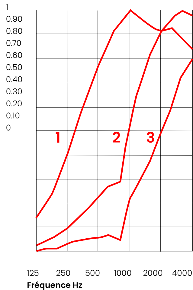
Coefficient d'absorption acoustique selon EN ISO 10534-2:2001
