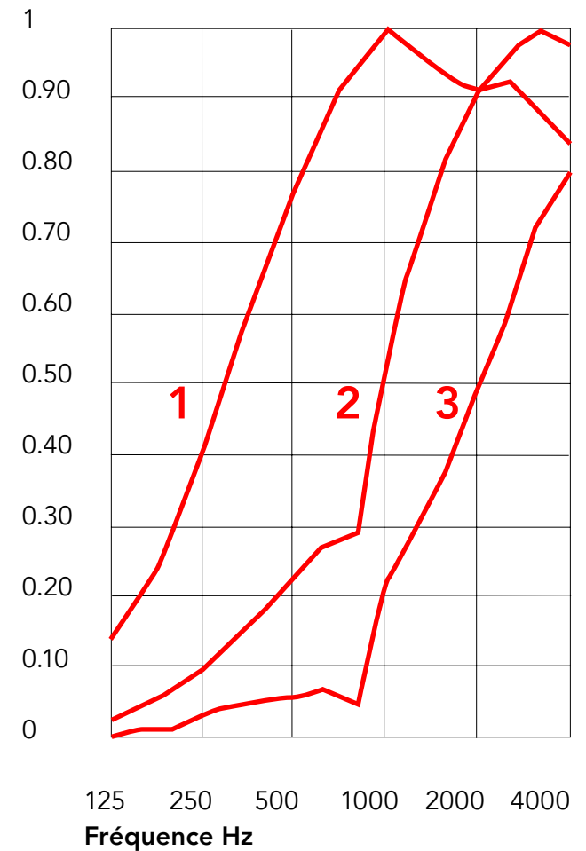
Coefficient d'absorption acoustique selon EN ISO 10534-2:2001
